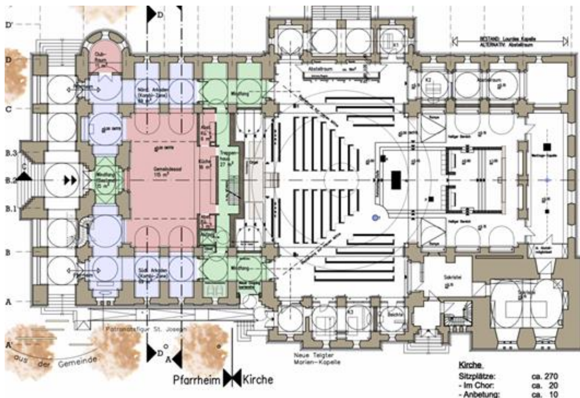
0-4: Umbauplan der Kirche St. Joseph in Osnabrück
