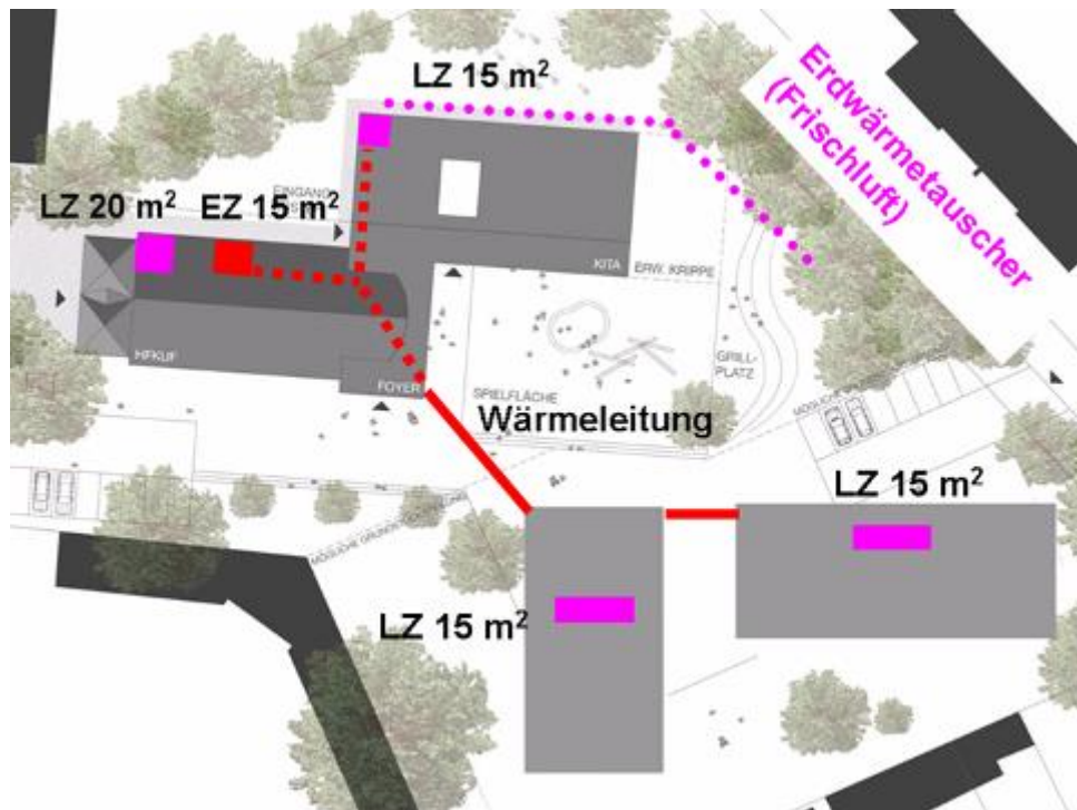
0-11: Lageplan der Gebäude der Kirchengemeinde St. Marien Bremen (Quelle: Planungsbüro Graw)
