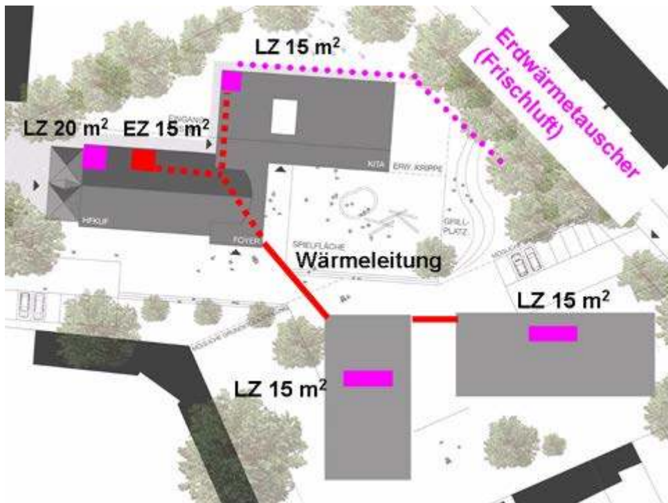
10-11: Lageplan der Gebäude der Kirchenburg St. Marien Bremen (Quelle: Planungsbüro Graw)
