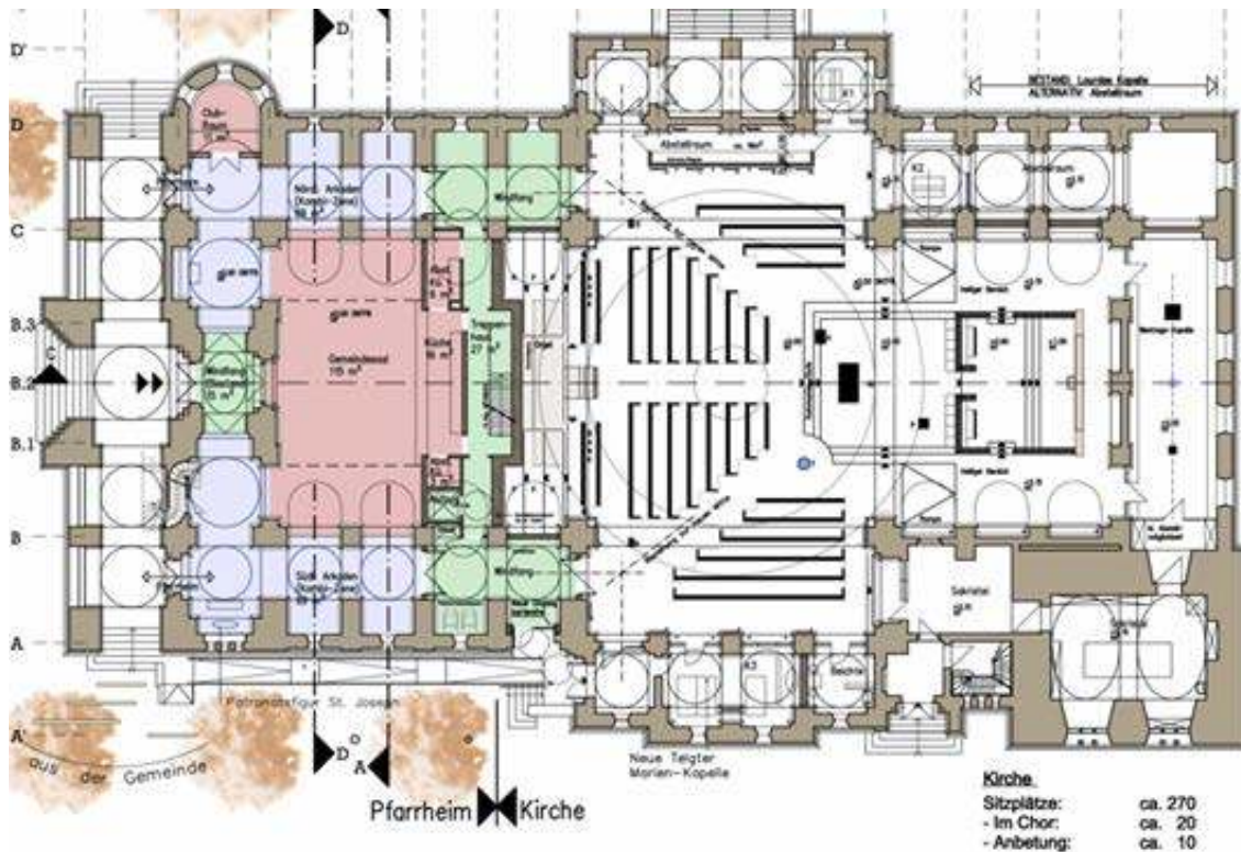
10-4: Umbauplan der Kirche St. Joseph in Osnabrück
